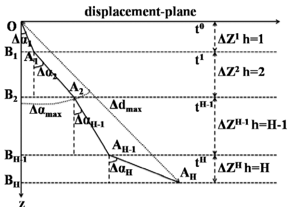
Fig. 14. Displacement-plane vs. depth.
