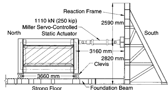
Fig. 6. Test setup
