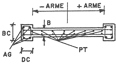
PLAN A-A
