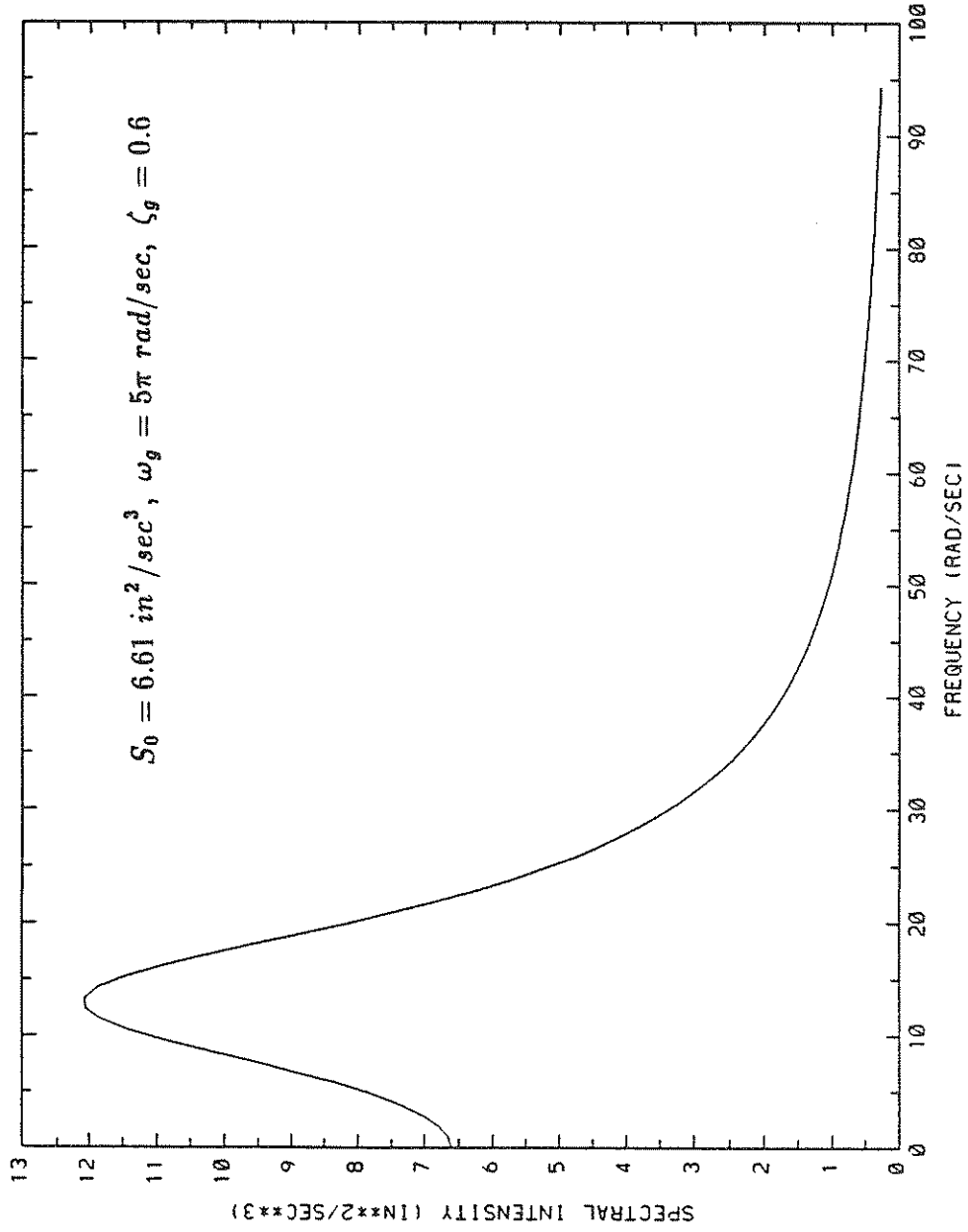
Fig. 6-3 Kanai-Tajimi Power Spectrum
